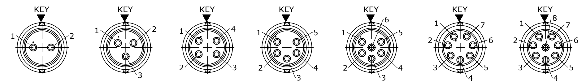
WIRING END W6282-2SG-P-3XX WIRING END W6282-3SG-P-3XX WIRING END W6282-4SG-P-3XX WIRING END W6282-5SG-P-3XX WIRING END W6282-6SG-P-3XX WIRING END W6282-7SG-P-3XX WIRING END W6282-8SG-P-3XX
