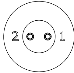
WIRING END ASSY: W7280-2PG-300
